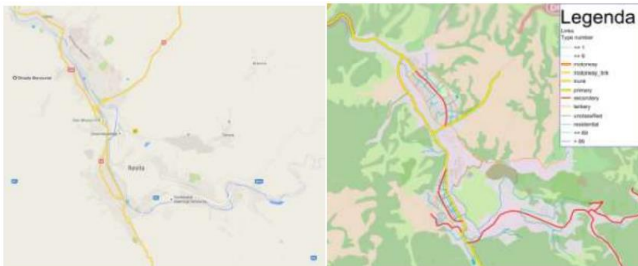
Figura 22: Rețeaua stradală
